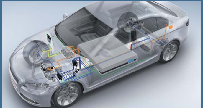
Elektrofahrzeug mit vakuum-unabhängigem regenerativen Bremssystem
