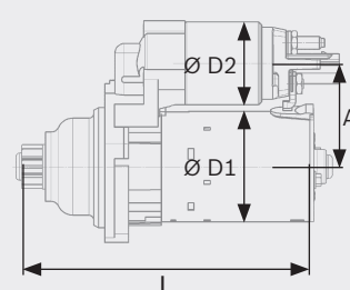
Freiausstoßender Starter
